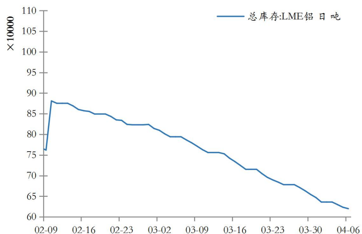
图 19: LME 铝库存单位: 吨
