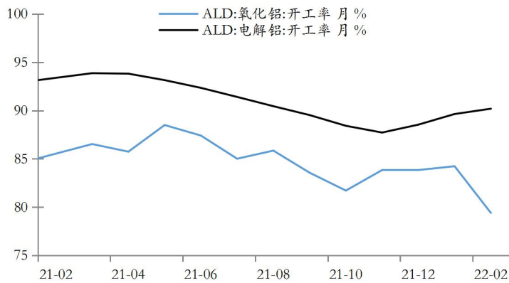
图 14：电解铝、氧化铝开工率单位：%
